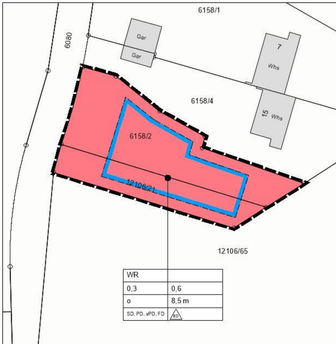
Abbildung 6.1: Bebauungsplan „Lortzingweg“
