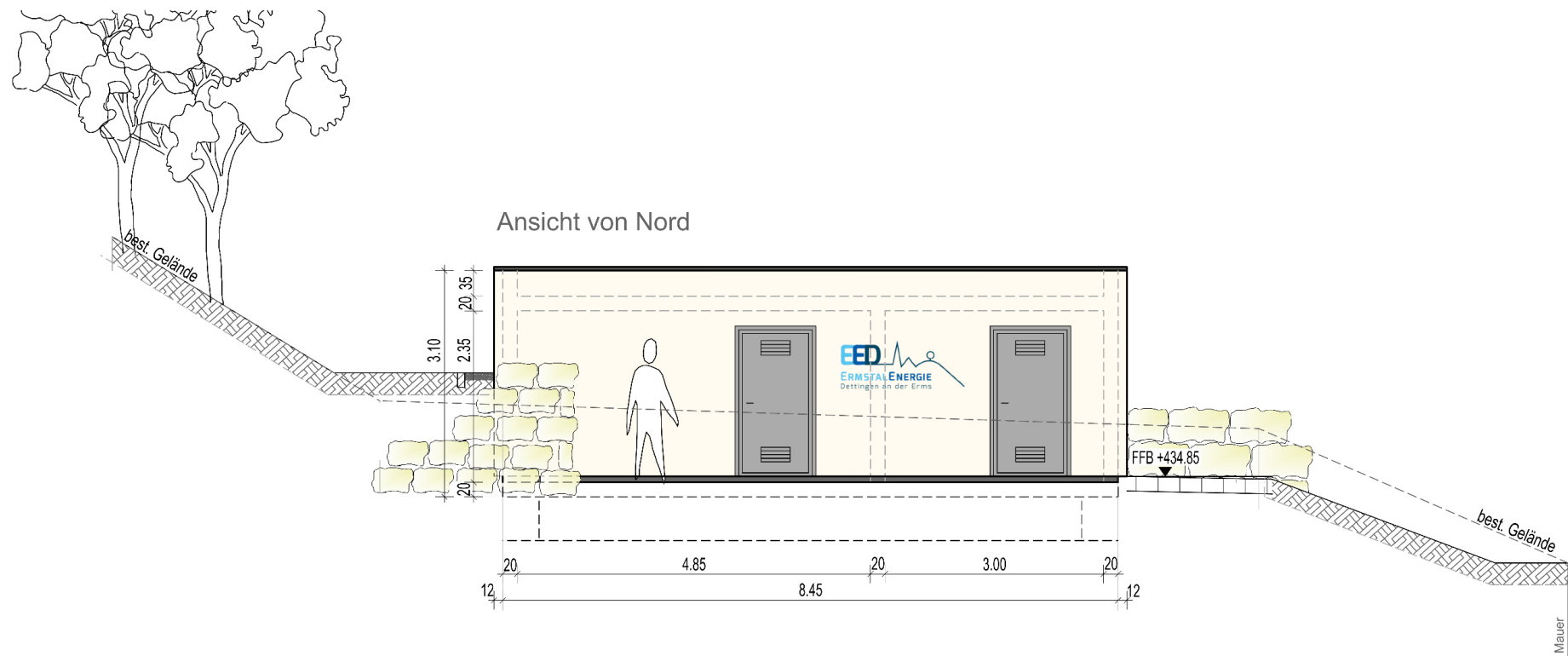
Abbildung 5.2: Ansicht des Zugangsbereichs von der Zufahrt aus (Ansicht von Norden aus), inkl. Darstellung des aktuellen und des Bestandsgeländes
