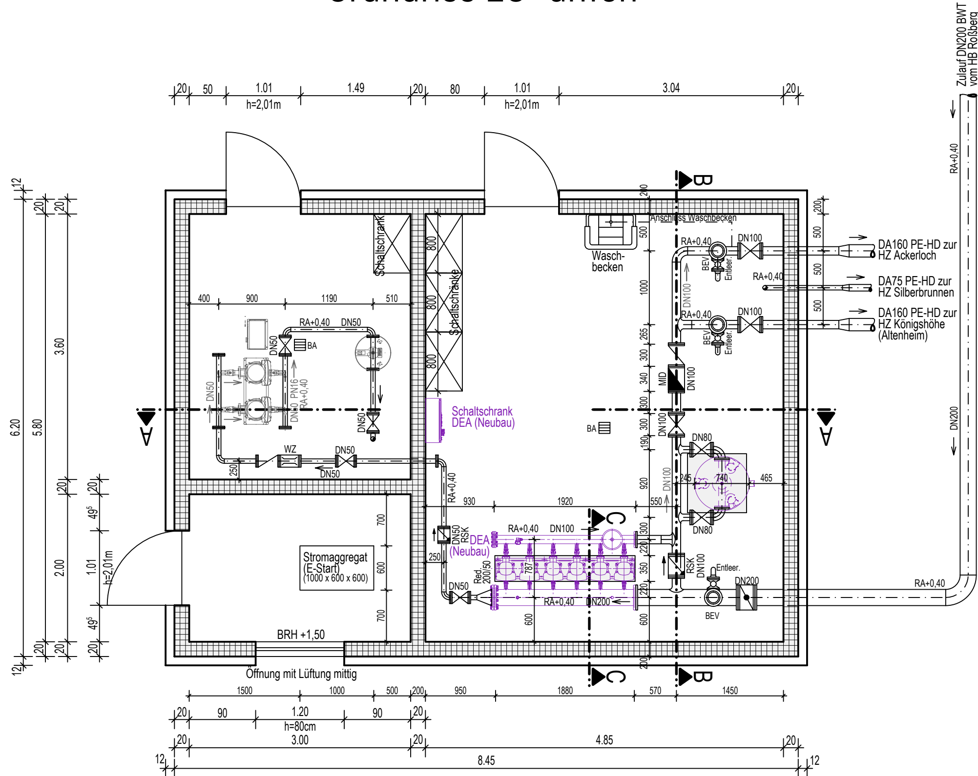
Grundriss EG "unten"
