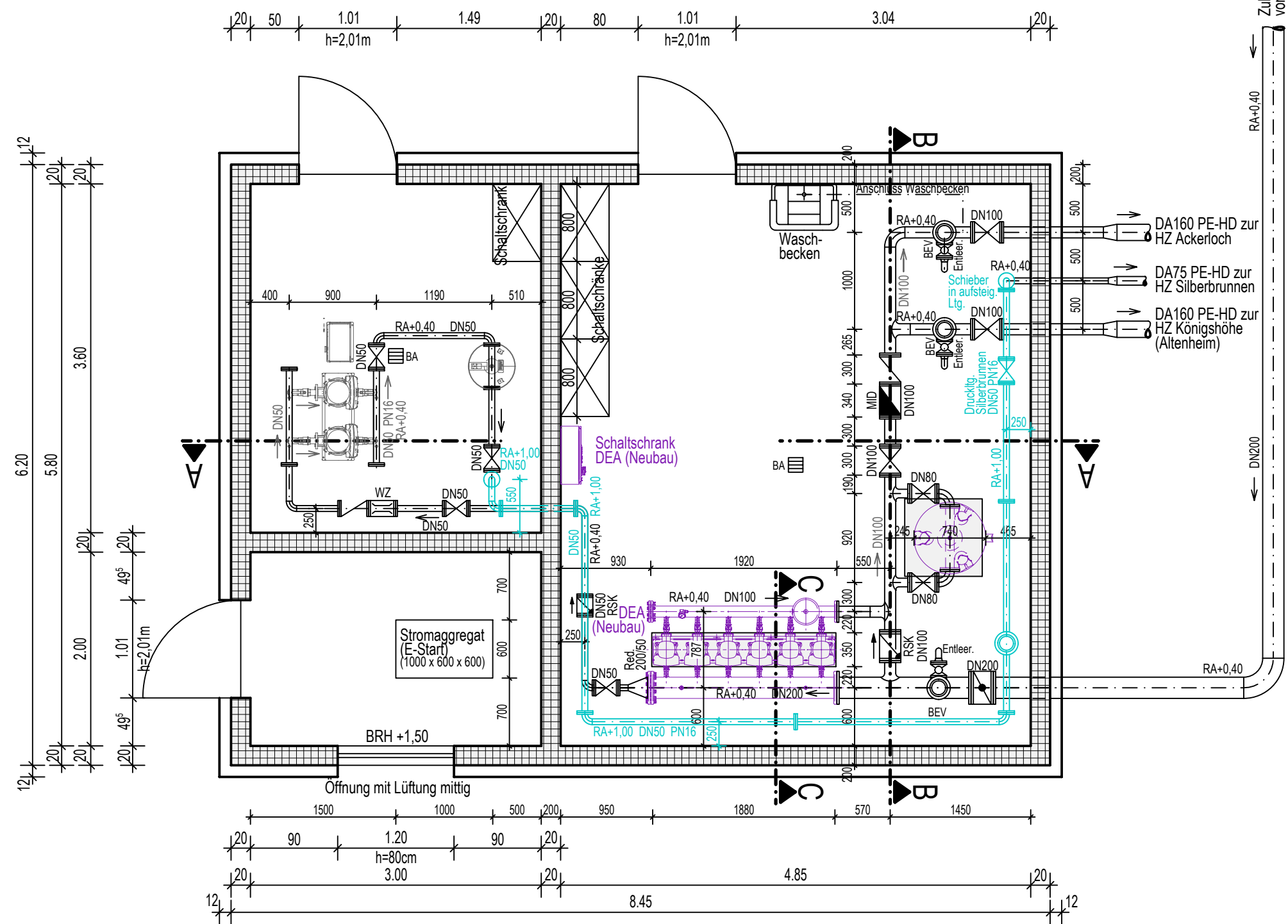
Grundriss EG "alles"
