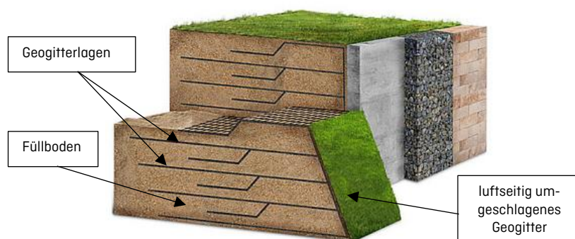
Abbildung 2.7: Ausführungsbeispiele für Bewehrte-Erde-Konstruktionen als Böschungssicherung: Fertige Konstruktion ohne Bewuchs (links), Herstellung und Verfüllung mit Bodenmaterial (rechts) und schematischer Aufbau (unten)
