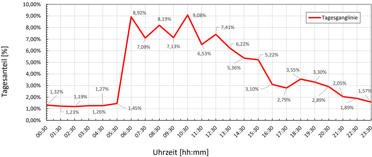
Normierte Tagesganglinie - HZ Ackerloch/Königshöhe
