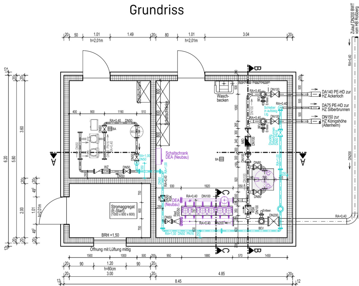
Abbildung 2.1: Grundriss des geplanten Pumpwerks mit hydraulischer Installation
