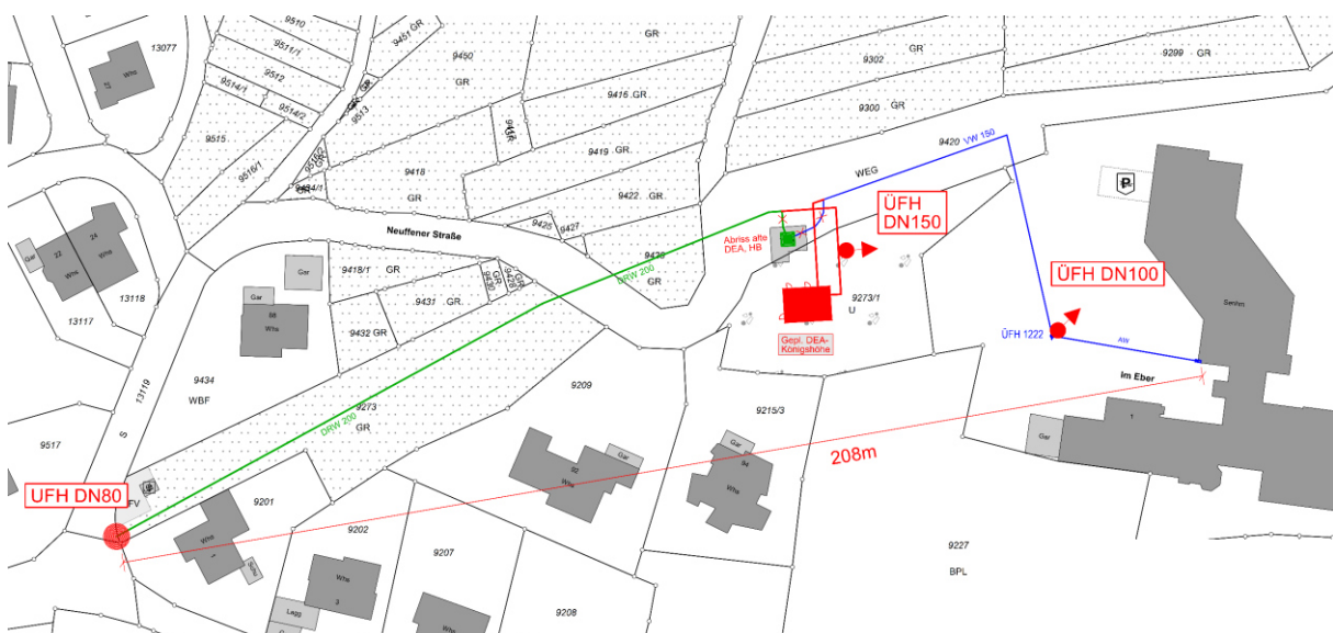
Abbildung 3.1: Lageplan zum Löschwasserkonzept des Pumpwerks Königshöhe
