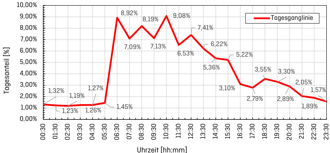
Abbildung 4.1: Normierte Tagesganglinie für das Versorgungsgebiete HZ Ackerloch/Königshöhe
