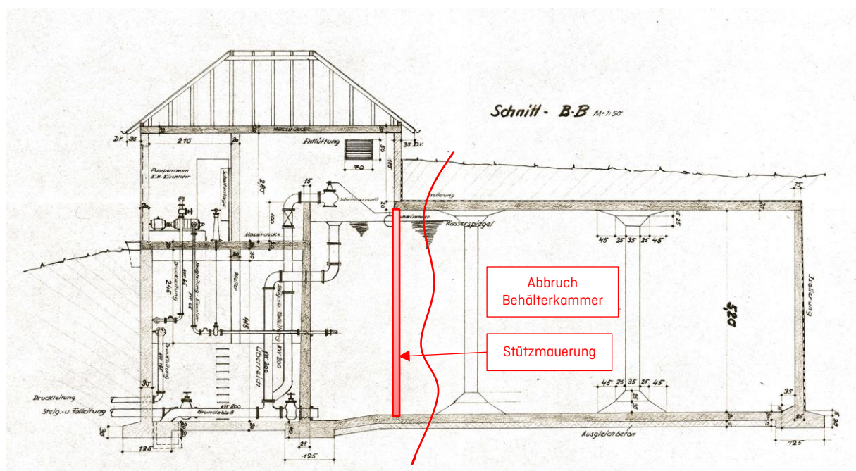
Abbildung 2.6: Abbruch Behälterkammer mit Stützmauerung
