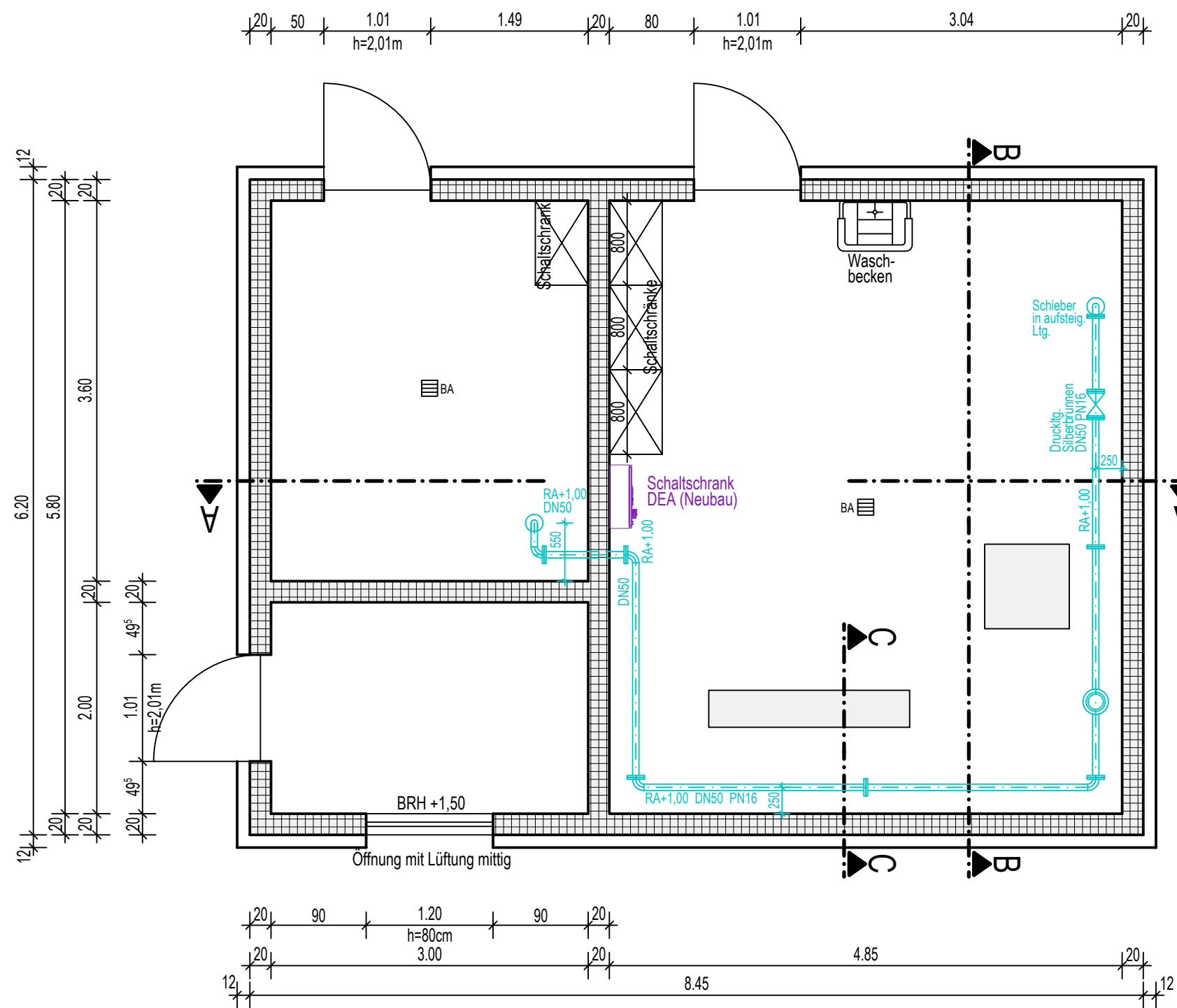
Grundriss EG "oben"
