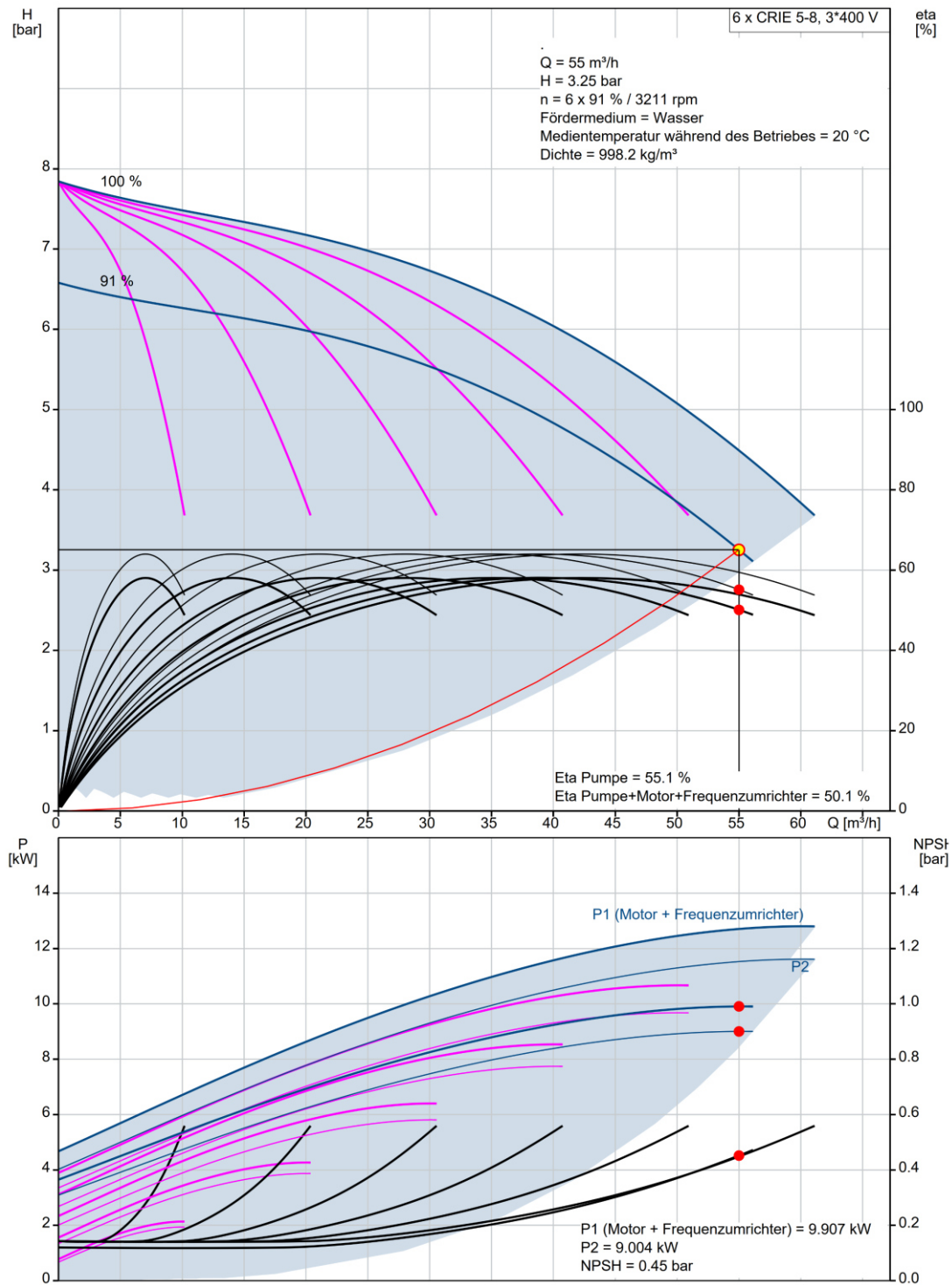
Abbildung 4.2: Auslegung der Druckerhöhungsanlage für den Lastfall des maßgebenden maximalbedarfs im Löschwasserfall Q_{FL,max} = 55 \text{ m}^3/\text{h} (gerundet) mit Angaben zum Wirkungsgrad und Leistungsbedarf
