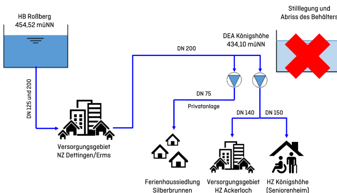
Abbildung 1.5: Versorgungsschema des neuen Pumpwerks
