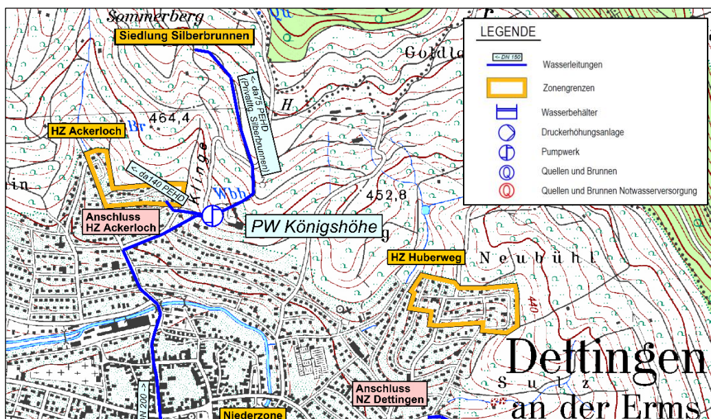
Abbildung 1.1: Lage und Einbindung PW Königshöhe
