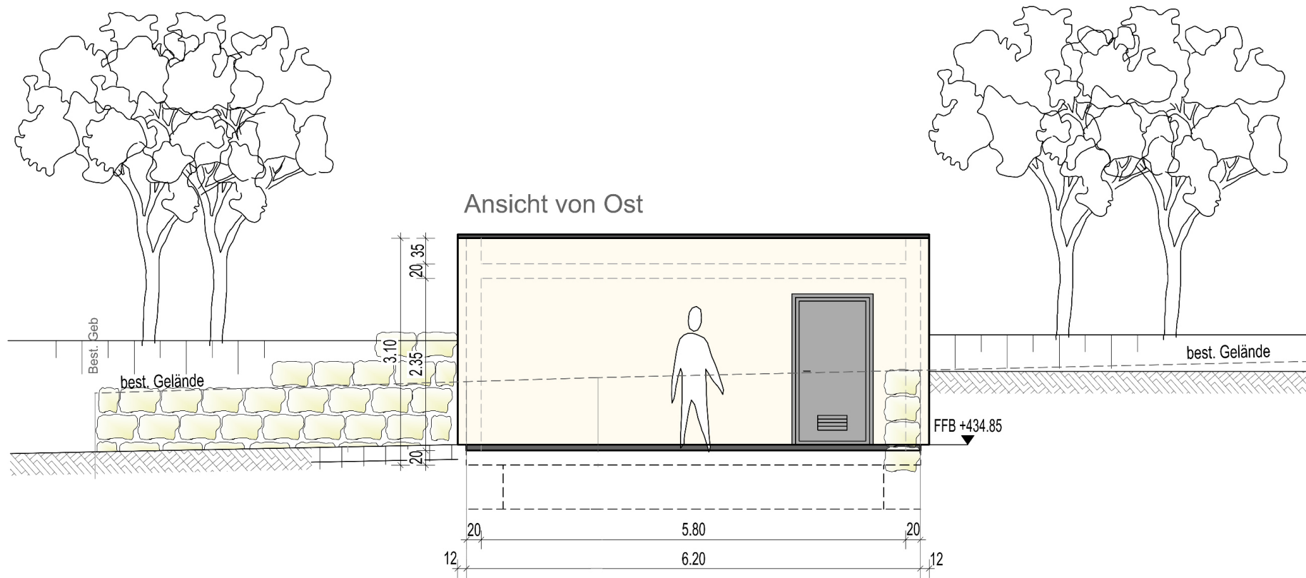
Abbildung 5.3: Ansicht der Eingangstüre für den Nebenraum in dem sich das Notstromaggregat befindet (Ansicht von Osten aus), inkl. Darstellung des aktuellen und des Bestandsgeländes
