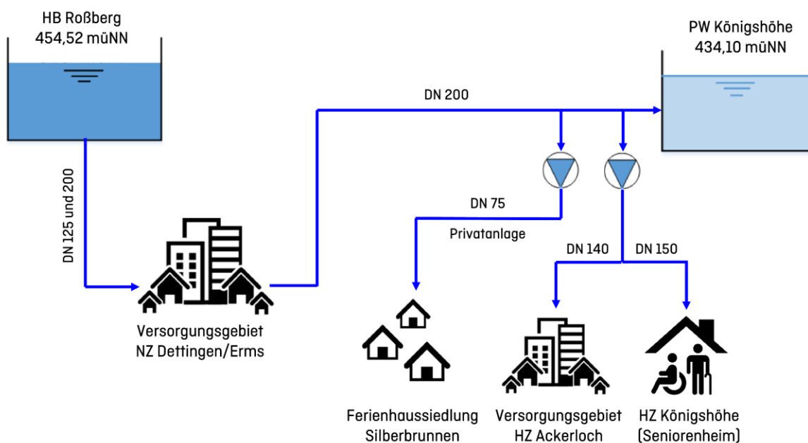
Abbildung 1.2: Aktuelles Versorgungsschema des Pumpwerks Königshöhe
