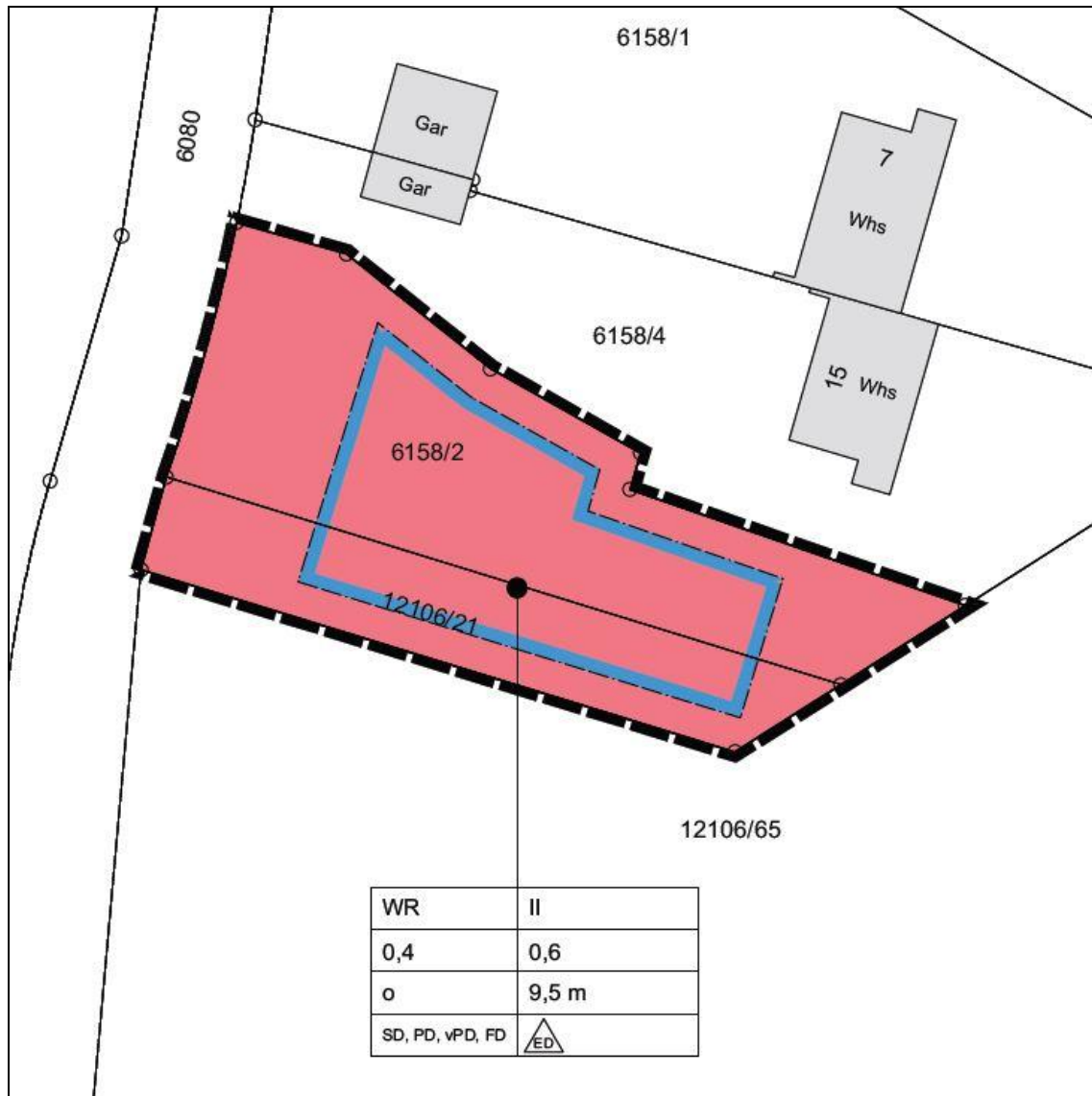
Abbildung 6.1: Bebauungsplan „Lortzingweg“
